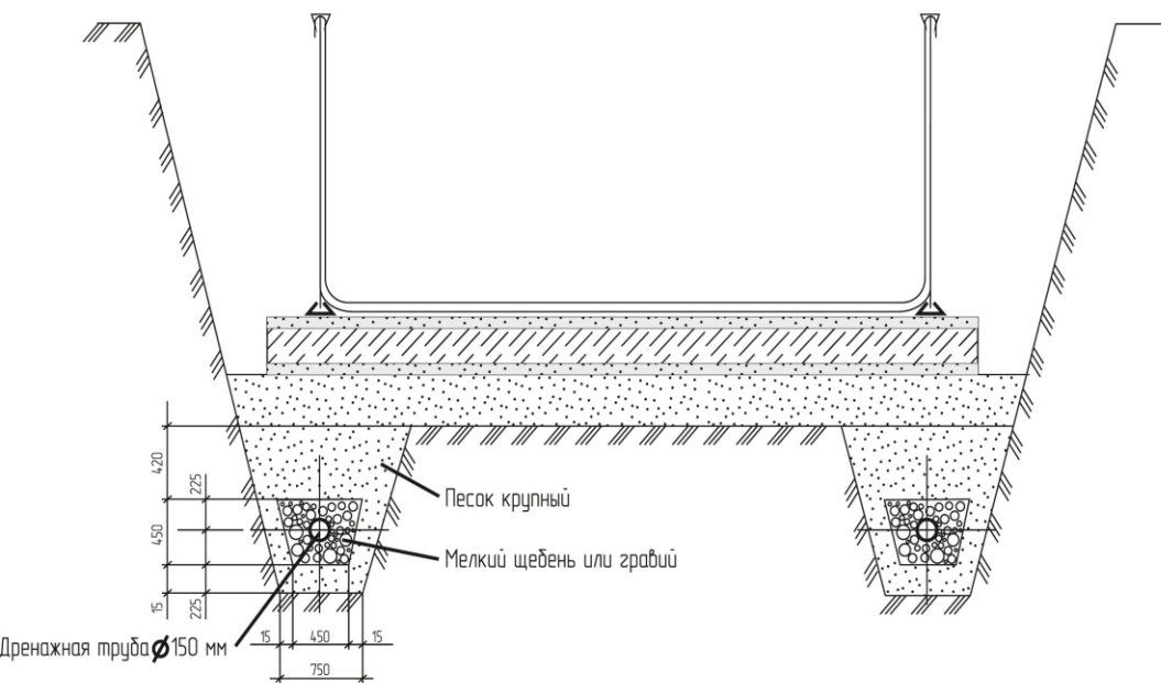
Рисунок №5. Схема устройства дренажа при наличии грунтовых вод
