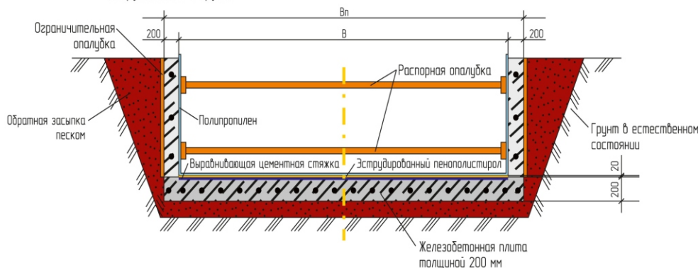
Рисунок №3. Схема устройства бассейна из полипропилена частично либо полностью погруженного в грунт.
